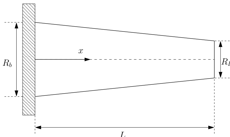
Figura 2: Vista lateral de uma aleta com formato de tronco de cone.
